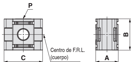
Tipo de cuerpo: estándar
