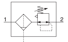
Función de flujo inverso
