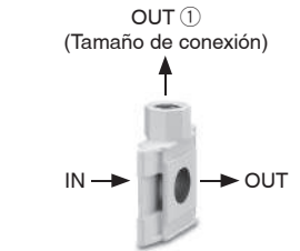
Tipo de cuerpo: diseño plano (Y□-□□-1-D)
