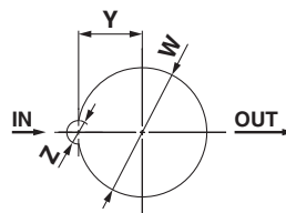
Dimensiones de montaje del panel
